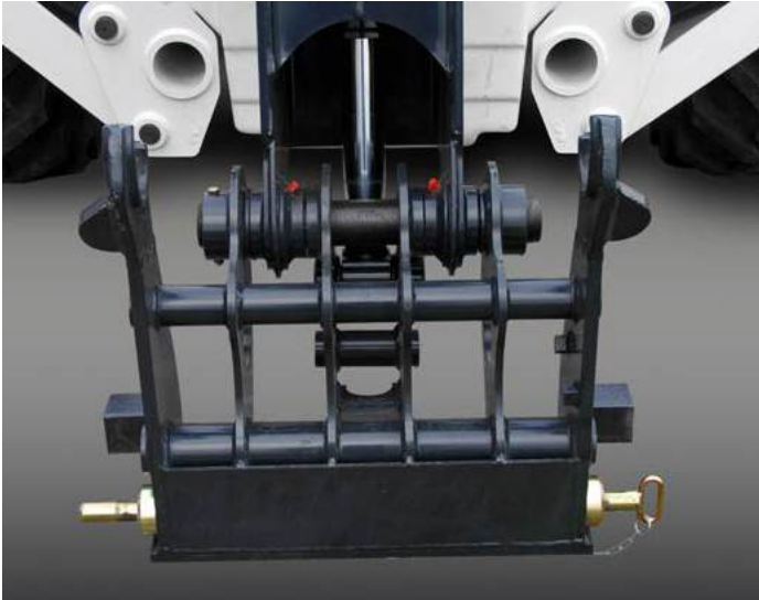
Manuelles Quick-Tach-System
